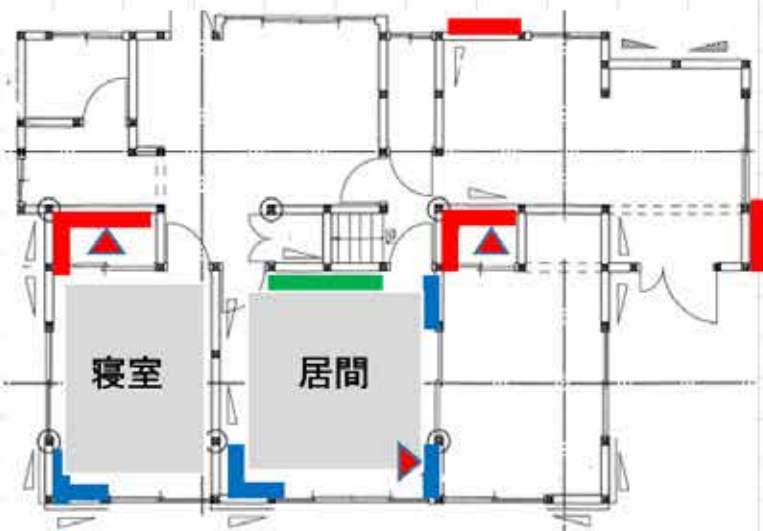
1階平面図
